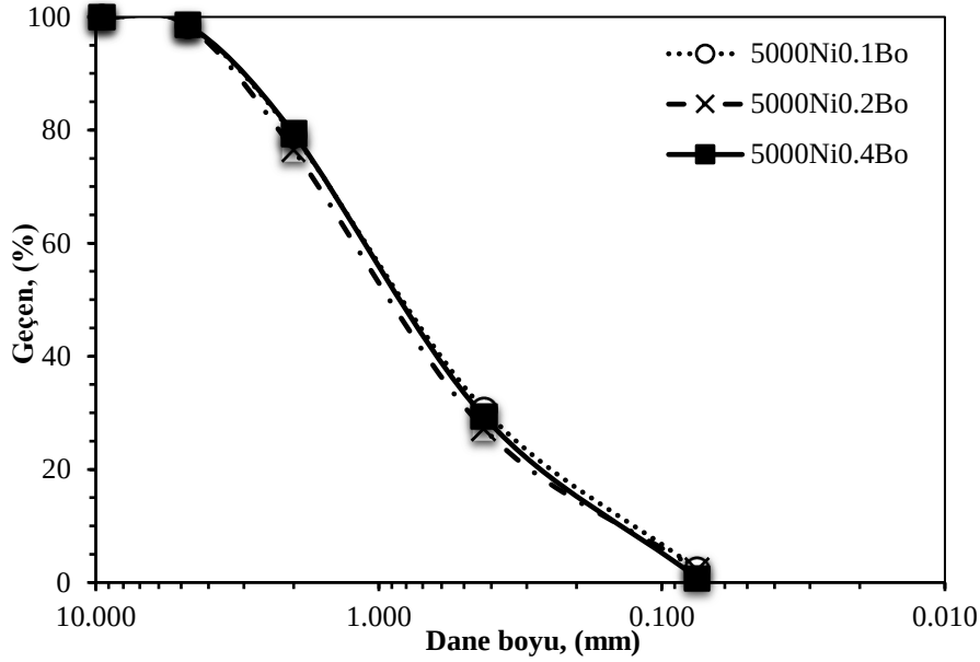
Görsel 5. 5000 ppm nikel sülfat ile kirlenilmiş numunelerin dane boyu dağılım eğrileri
