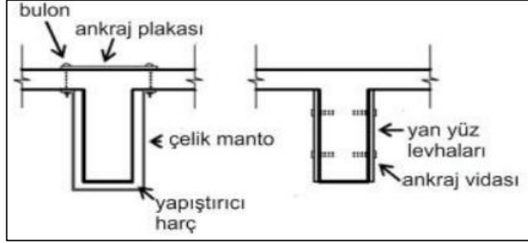
Görsel 4.2 Çelik levhalar ile kiriş güçlendirmesine ait detay örnekleri (Özdemir & Ercan,2017).
