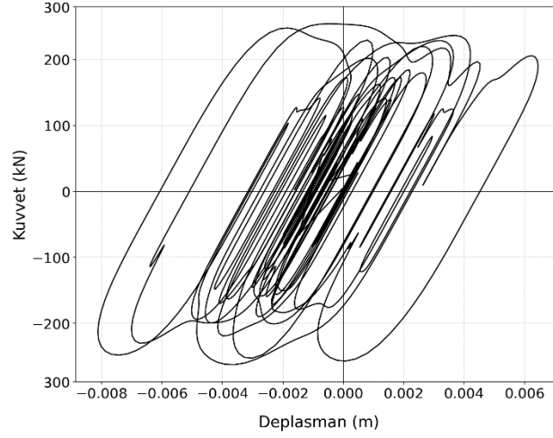
Görsel 8. VAS (Nominal Kuvvet 500 kN) için Kuvvet-Yerdeğiştirme Sonuçları
