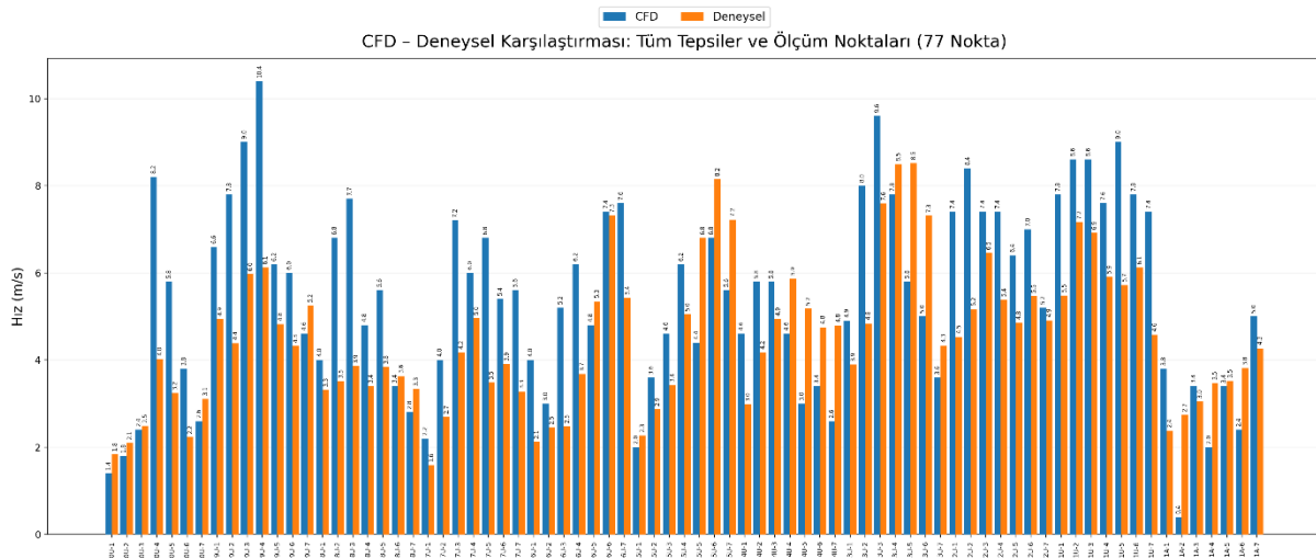
Görsel 9. Tüm Tepsiler ve Ölçüm Noktaları için CFD-Deneysel Karşılaştırması
