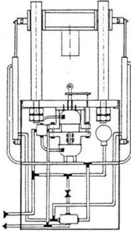
Görsel 2.1. Yorulma test cihazının genel görünüşü [5]
