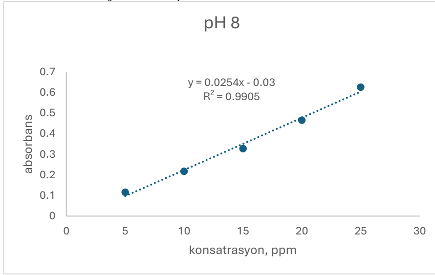
Görsel 3. pH kalibrasyon grafiği
