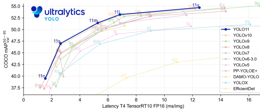
Görsel 3. Yolo versiyonlarının hız-doğruluk dengesi [23]
