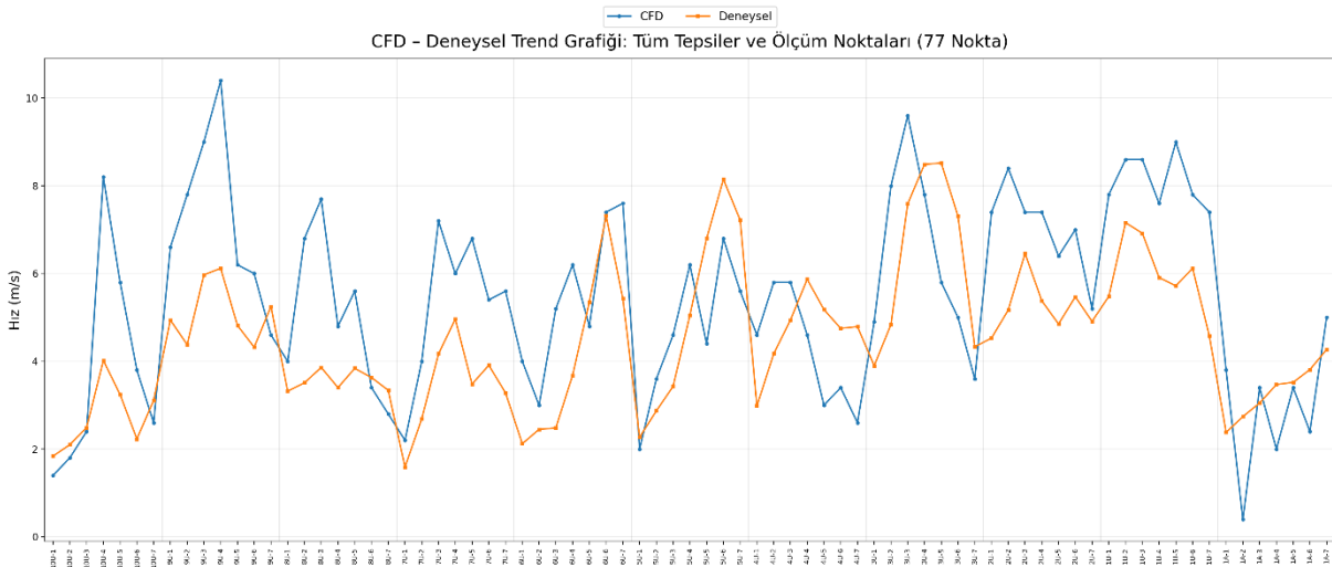
Görsel 11. Tüm Tepsiler ve Ölçüm Noktaları için CFD-Deneysel Trend Grafiği
