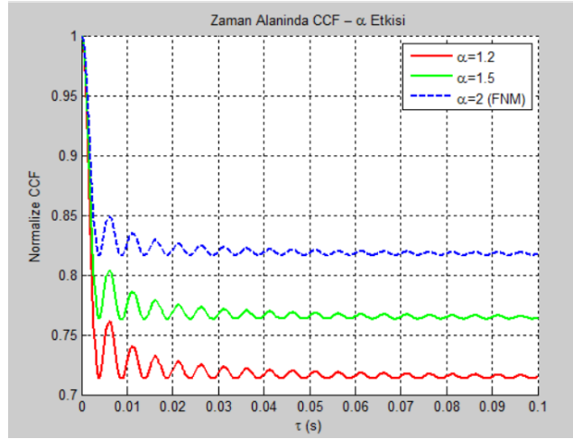
Görsel 1. Zaman Alanı Çapraz İlinti Fonksiyonu Grafiği
