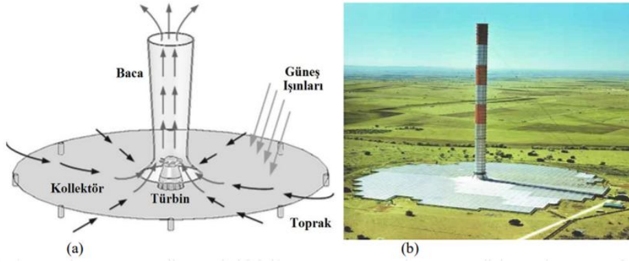
Görsel 5. a) Şematik Güneş Bacası, b) Manzaranes Güneş Bacası, İspanya (Köse, 2018)
