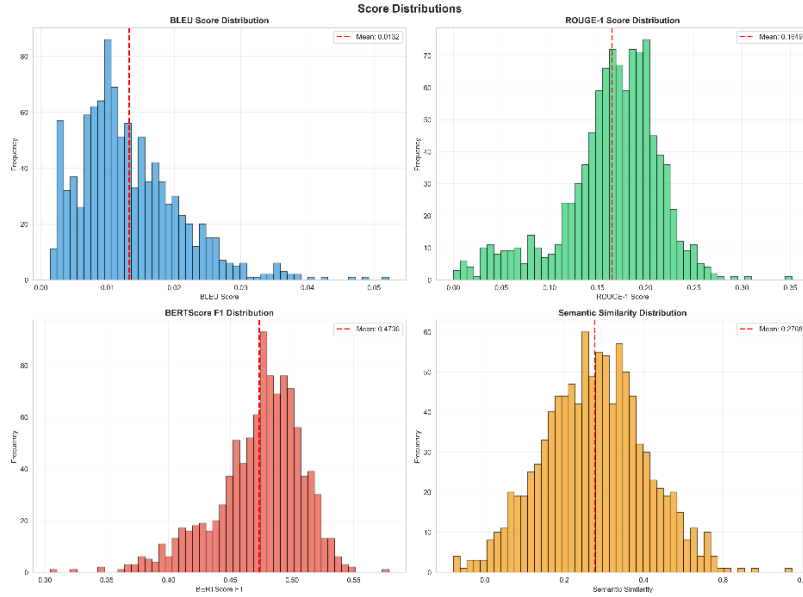
Görsel 2. QLoRA tabanlı ince ayar sonrası model çıktılarının farklı değerlendirme metrikleri açısından skor dağılımları
