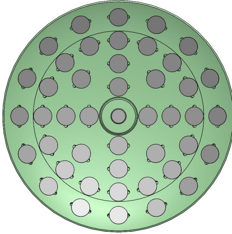
Görsel 3. Kaplin sistem mıknatıs PTFE kapak yerleşim
