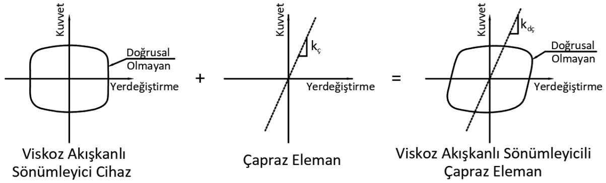
Görsel 6. VAS için İdealize Edilmiş Kuvvet–Yerdeğiştirme İlişkileri [16,35]
