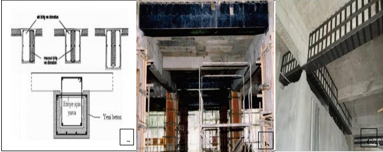
Görsel 4 a. Betonarme kiriş mantosu detayı(Özdemir & Ercan 2017). B. Kiriş mantolaması 2 . c. Yatay kiriş mantolama yöntemi 3 .
