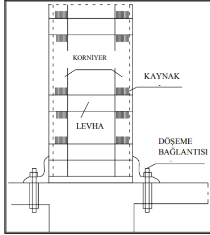
Görsel 7. Betonarme kolonda çelik mantolama uygulaması (Demirkan, 2014).
