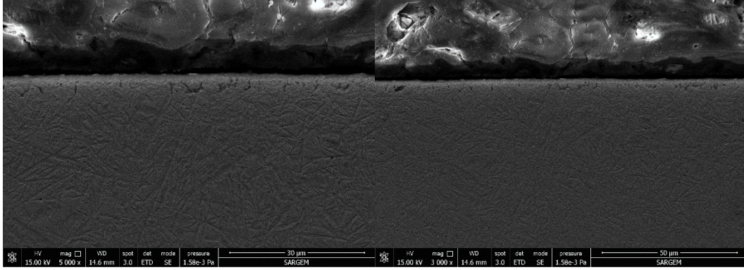
Görsel 3.7. Karbonitrürleme işlemi sonucu elde edilen SEM görüntüleri.
