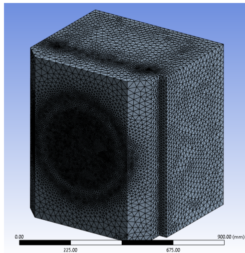
Görsel 5. 36 Milyon Hücreli Ağ (Mesh) Yapısı
