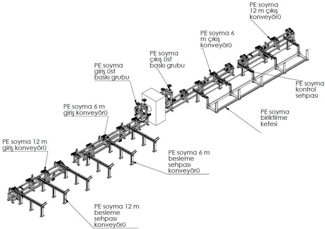
Görsel 1. Mekanik Tel Fırça Tabanlı Sıyırma Sistemi 3B çizimi.
