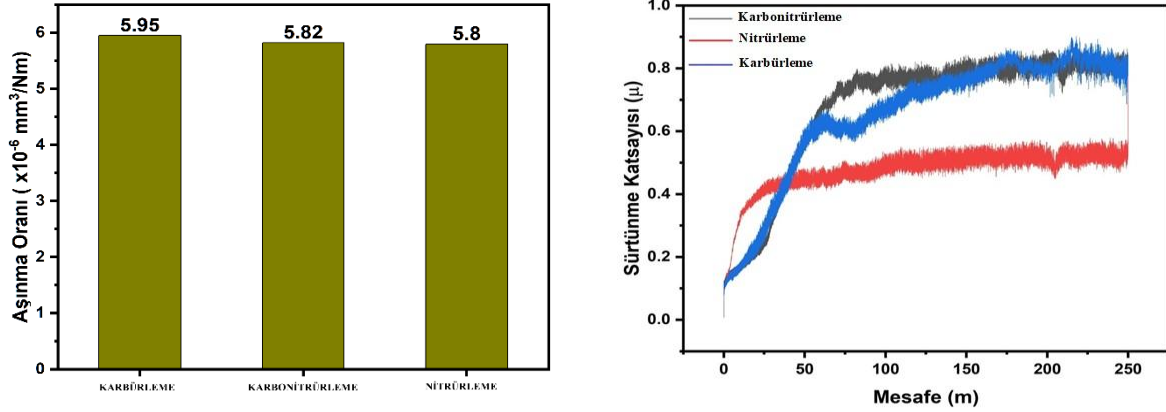
Görsel 3.11. Numunelere ait aşınma oranı ve sürtünme katsayı değerleri.
