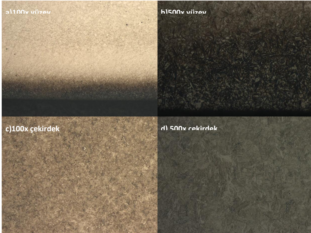
Görsel 3.4. Karbonitrüleme a)100x yüzey b)500x yüzey, c)100x çekirdek d)500x çekirdek
