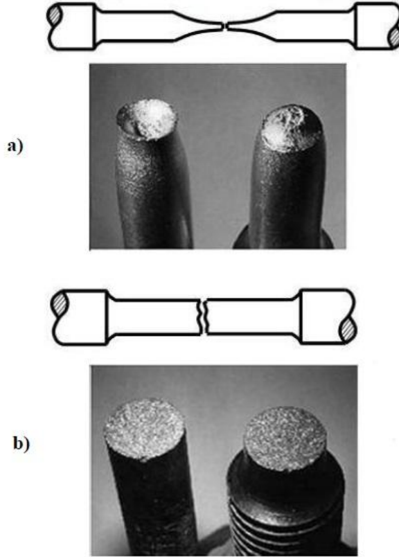
Görsel 2.1. a) Sünek malzeme b) Gevrek malzeme [1]
