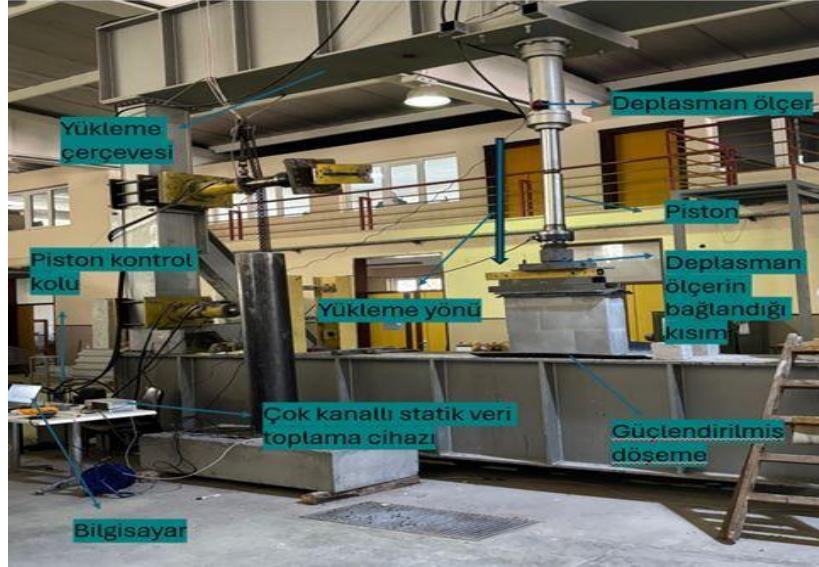
Görsel 3 Yüklem çerçevesi
