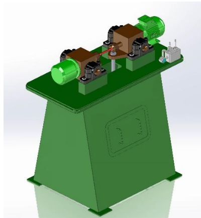
Görsel 3.1. Döner eğmeli yorulma test cihazı tasarımı 3B görünüş
