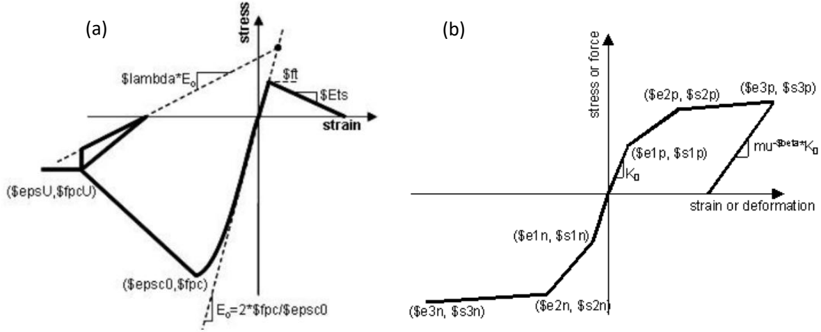
Görsel 2. “Concrete02” ve “uniaxialMaterial” Malzeme Modellerine ait Gerilme–Şekil Değiştirme İlişkileri
