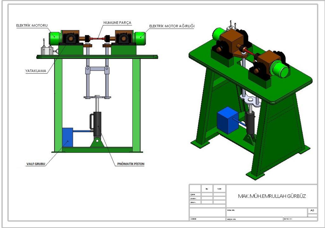
Görsel 3.2. Döner eğmeli yorulma test cihazı tasarımı ön görünüş
