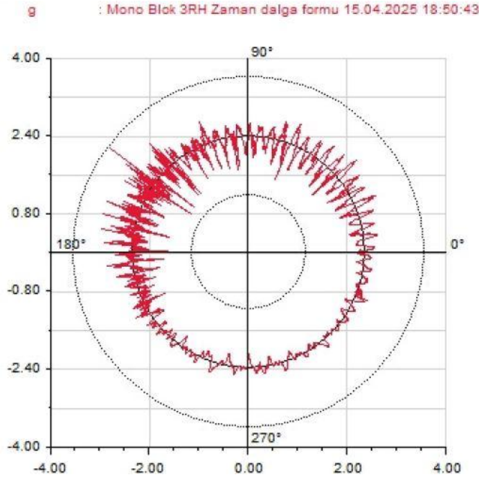
Görsel 3. Titreşim Analizi Zaman Dalga Form Grafiği.
