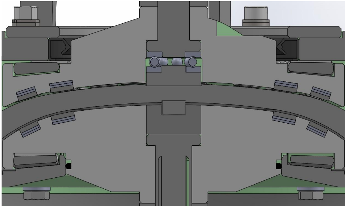
Görsel 1. Kaplin sistem montaj örneği
