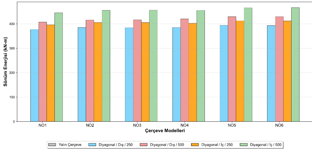
Görsel 12. 15 Katlı Çerçevelerin Sönüm Enerji Grafiği
