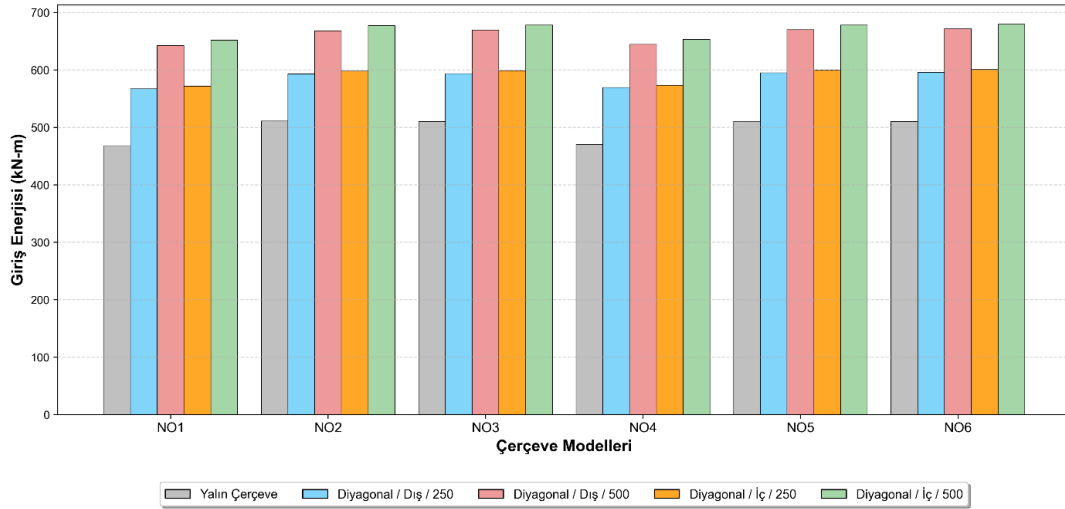
Görsel 11. 15 Katlı Çerçevelerin Deprem Giriş Enerji Grafiği
