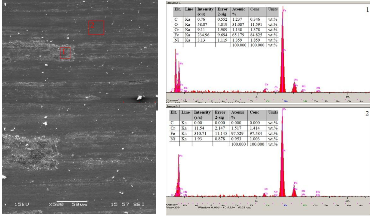
Görsel 3.13. Karbonitrürlenmiş numunenin aşınma sonrası SEM ve EDS analizleri.
