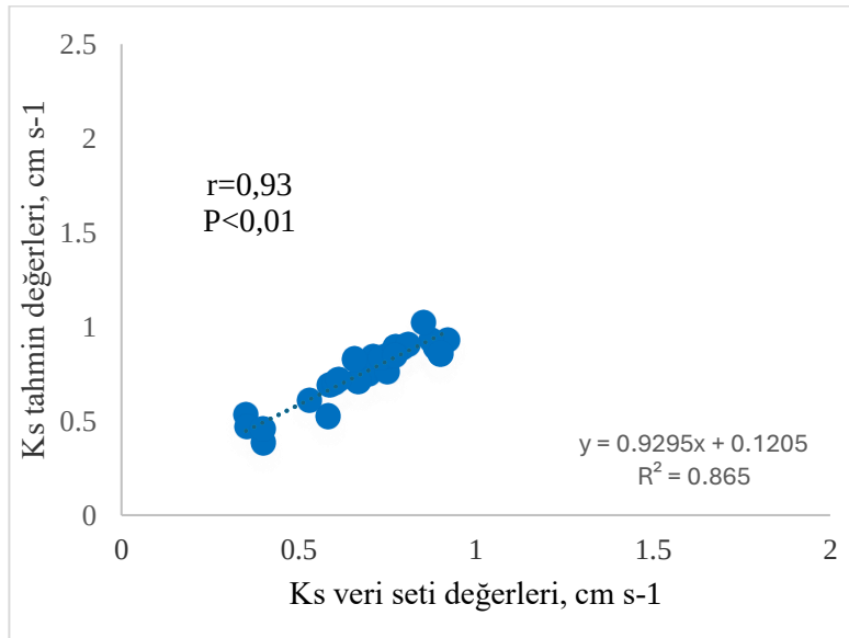
Görsel 4. Veri seti ölçülen ve tahmin edilen K_s değerleri arasındaki ilişki
