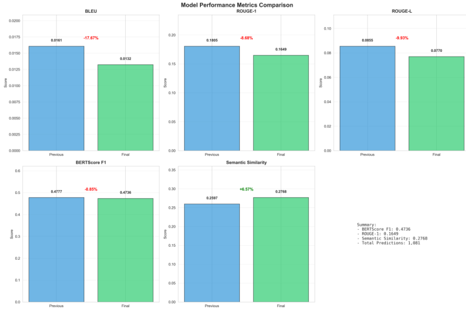
Görsel 1. QLoRA tabanlı ince ayar sonrası model performansının farklı değerlendirme metrikleri açısından karşılaştırılması
