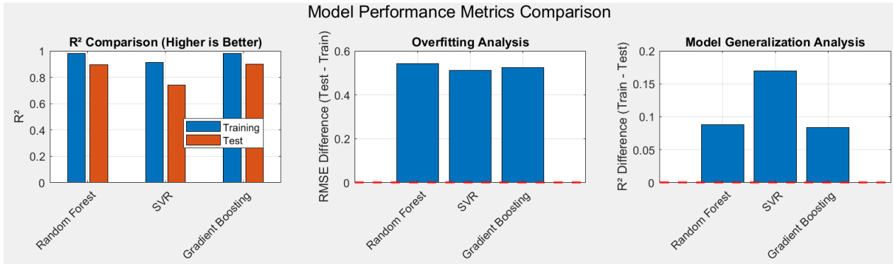
Görsel 2. Model Performansları
