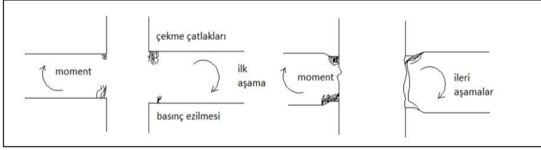
Görsel 1. Deprem etkisi altında kirişlerde moment hasarı (Koç, 2005)
