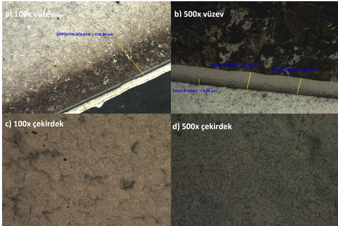
Görsel 3.5. Nitrürleme a)100x yüzey, b)500x yüzey, c)100x çekirdek, d)500x çekirdek
