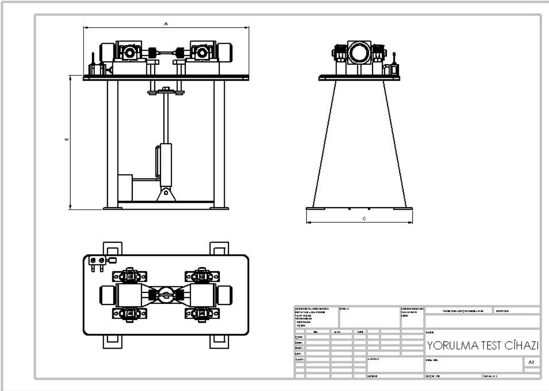
Görsel 3.3. Döner eğmeli yorulma test cihazı tasarımı üç görünüş
