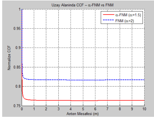
Görsel 3. Uzay Alanı Çapraz İlinti Fonksiyonu Grafiği
