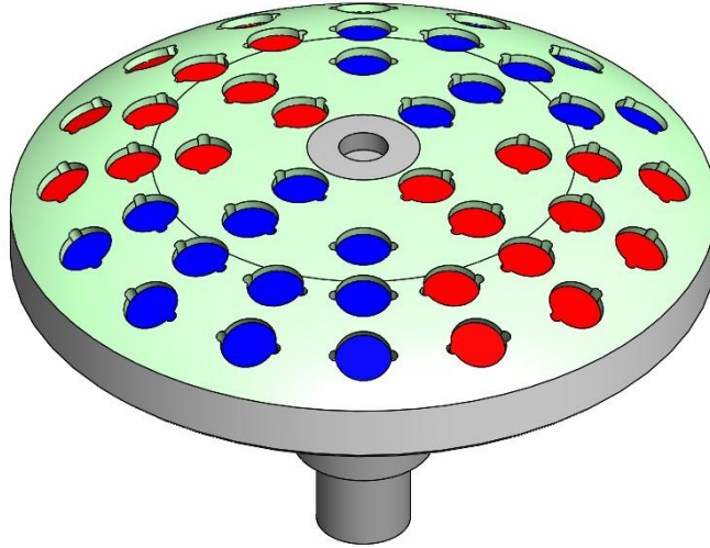
Görsel 2. Kaplin sistem mıknatıs yerleşim
