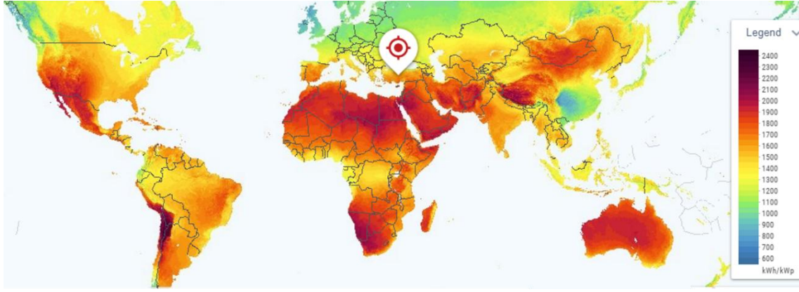
Görsel 15. Küresel çapta spesifik fotovoltaik güç çıkışları
