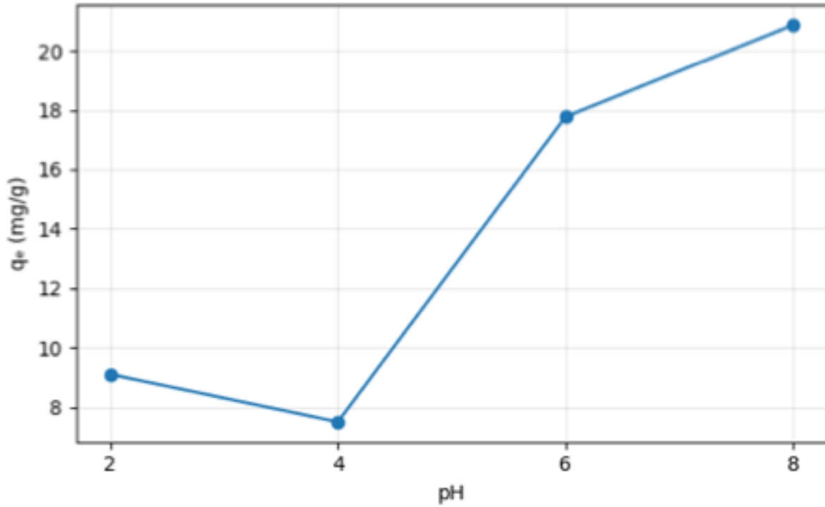
Görsel 5. pH- Q_e grafiği
