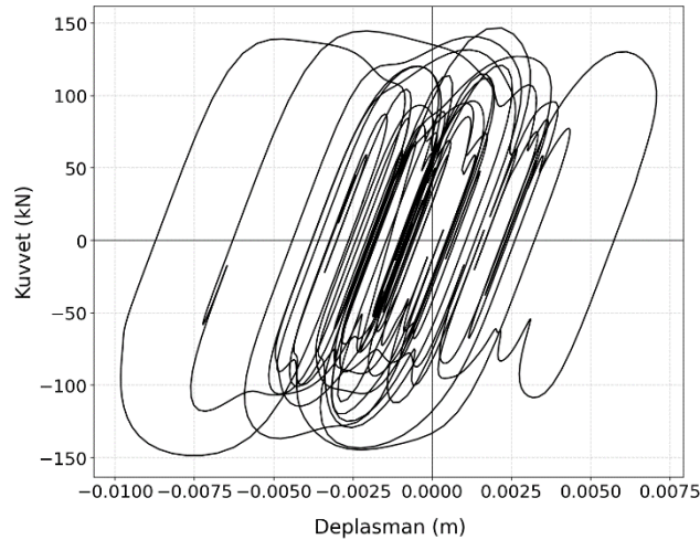
Görsel 7. VAS (Nominal Kuvvet 250 kN) için Kuvvet–Deplasman Sonuçları
