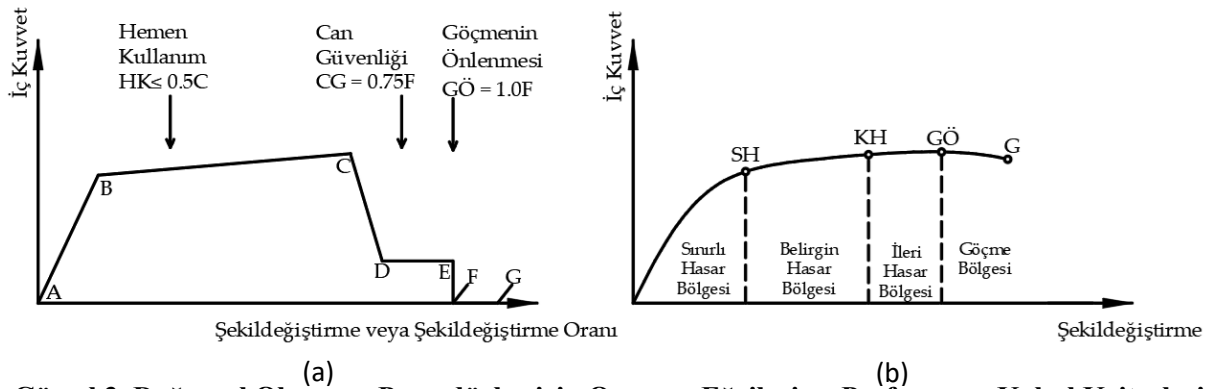
Görsel 3. Doğrusal Olmayan Prosedürler için Omurga Eğrileri ve Performans Kabul Kriterleri
