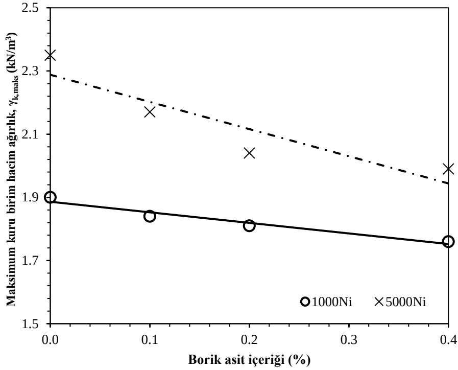
Görsel 9. Borik asit remedasyonunun farklı nikel konsantrasyonlarında maksimum kuru birim hacim ağırlık üzerindeki etkisi
