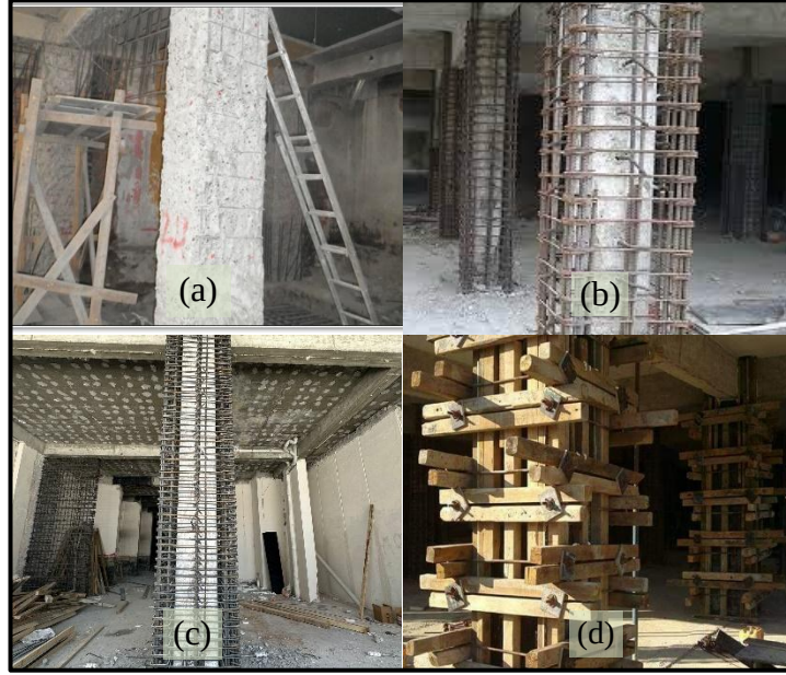
Görsel 6. Kolonda mantolama uygulamaları (URL 5) a) Mantolama için eski betonun yüzeyi pürüzlendirme, b,c) donatı yerleştirme, ankraj yapılma ve d) kalıp çakılması.
