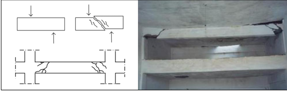
Görsel 3. Kirişte oluşabilecek kırılma çatlaklar (Yılmaz & Umut, 2017)
