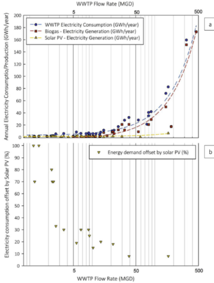
Görsel 24. a) AAT'de elektrik tüketimi (mavi), biyogazdan elektrik üretimi (kırmızı), güneş FV'den elektrik üretimi (sarı) b) FV ile dengelenen elektrik tüketimi
