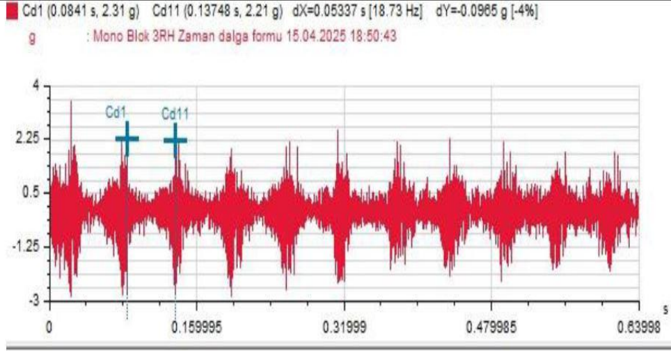
Görsel 2. Kangal Hattı Monoblok Titreşim Analizi Grafiği.
