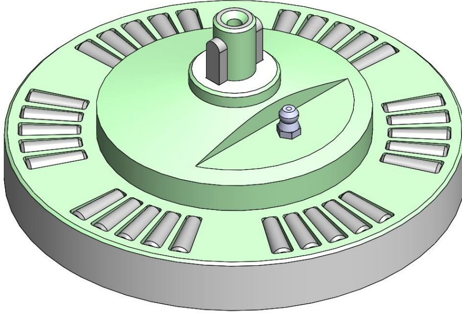
Görsel 4. Kaplin sistem PTFE masura yerleşim
