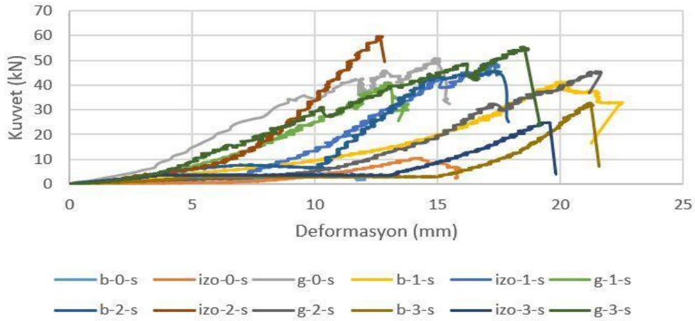
Görsel 9 Diagonal yükleme karşılaştırma grafiği
