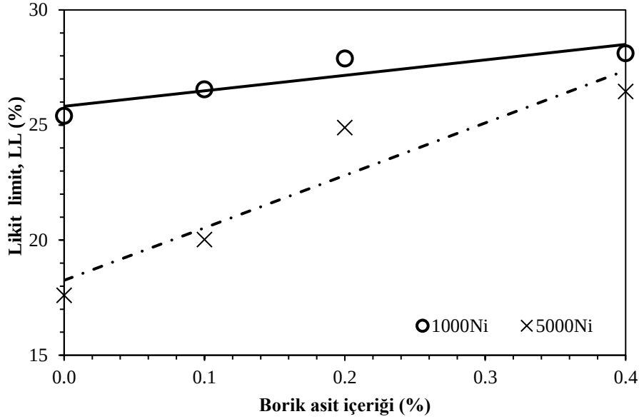
Görsel 8. Borik asit remedasyonunun farklı nikel konsantrasyonlarında likit limit üzerindeki etkisi
