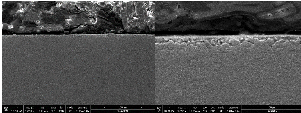
Görsel 3.6 Karbürleme işlemi sonucu elde edilen SEM görüntüleri.
