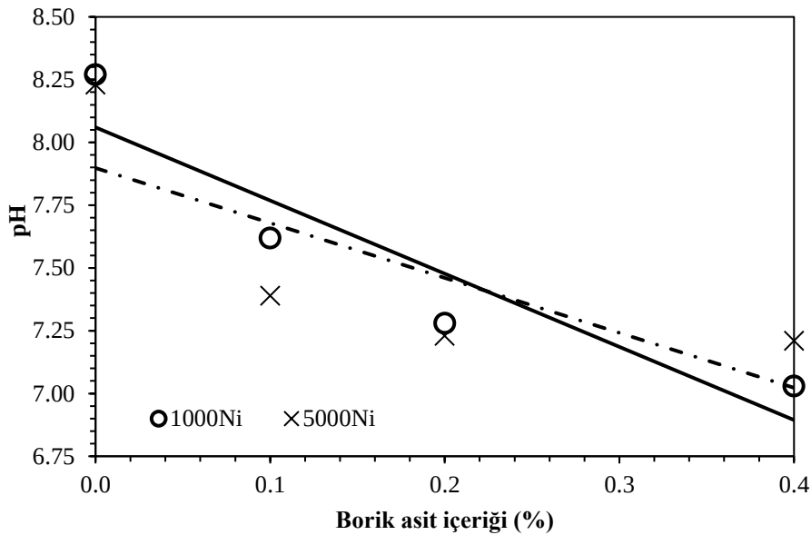
Görsel 11. Borik asit remedasyonunun farklı nikel konsantrasyonlarında pH üzerindeki etkisi
