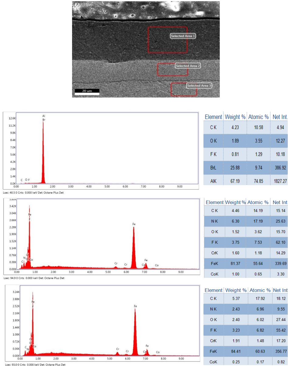
Görsel 3.10. EDS analizi noktaları ve sonuçları
