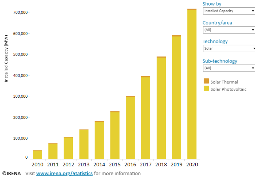
Görsel 16. Dünya çapında güneş enerjisinden faydalanılan teknolojilerin kurulu gücünün yıllara göre değişimi
