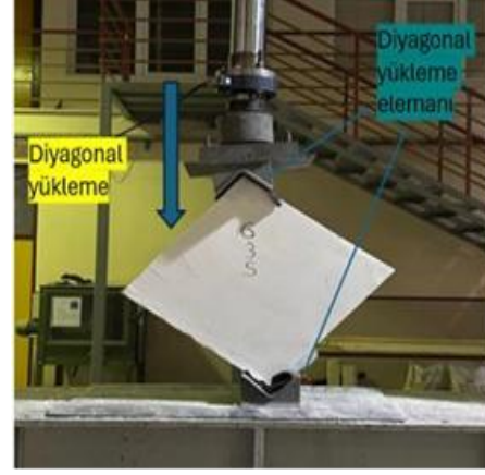
(b) Diyagonal yönde yükleme örneği
