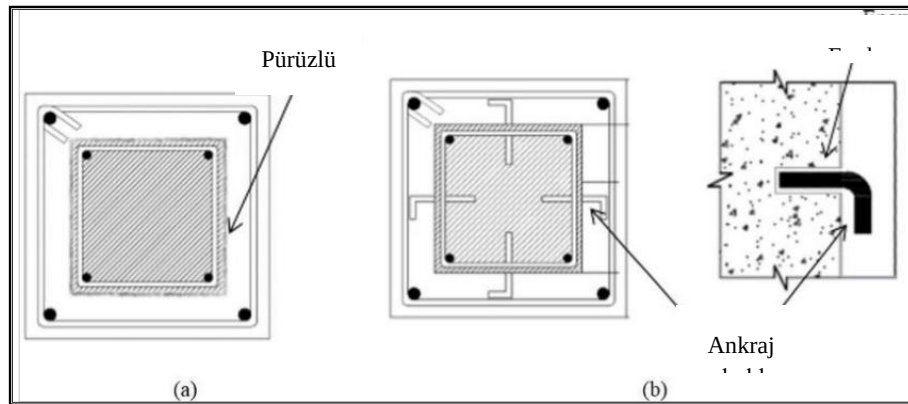
Görsel 4. Mantolanmış kolonun a) Yüzeyi pürüzlendirilme ve b) Ankraj yapılma şekli (Caglar ve ark., 2020).
