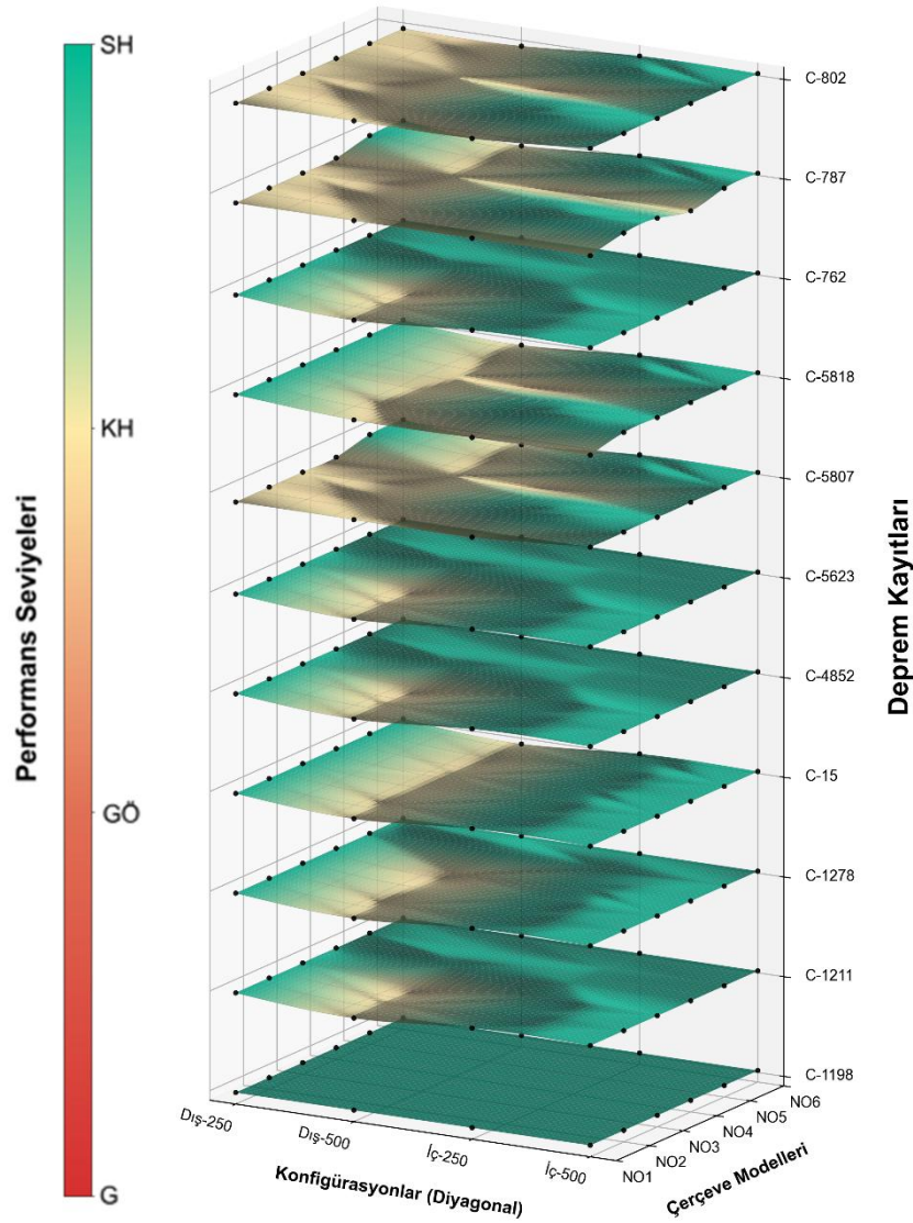
Görsel 14. 15 Katlı Çerçeveler için Deprem Performans Esaslı Öneri Grafiği
