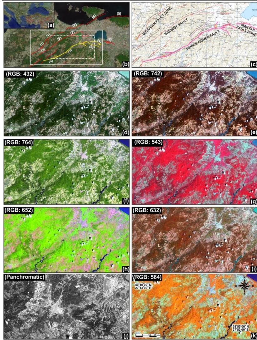
Şekil 3. (a) Türkiye'nin aktif tektonik unsurları üzerinde çalışma alanının gösterimi (Emre ve diğ., 2011a, 2011b, 2013) (b) Kesikli çizgi ile gösterilen çalışma alanında yer alan önemli aktif tektonik yapılar (Emre ve diğ., 2011a, 2011b, 2013) (1:Biga-Çan Fay Zonu, 2:Sarıköy Fayı, 3:Yenice-Gönen Fayı) (c) Diri Fay haritası üzerinde çalışma alanı içerisinde yer alan aktif faylar (Emre ve diğ., 2011a, 2011b, 2013) (d-i) Çalışma alanına ait LANDSAT8-OLI uydu görüntüsü ile denenen çeşitli bant kombinasyonları ile oluşturulan görüntüler. (j) Pankromatik band (Band:8) (k) Tercih edilen band kombinasyonu (RGB: 564)
