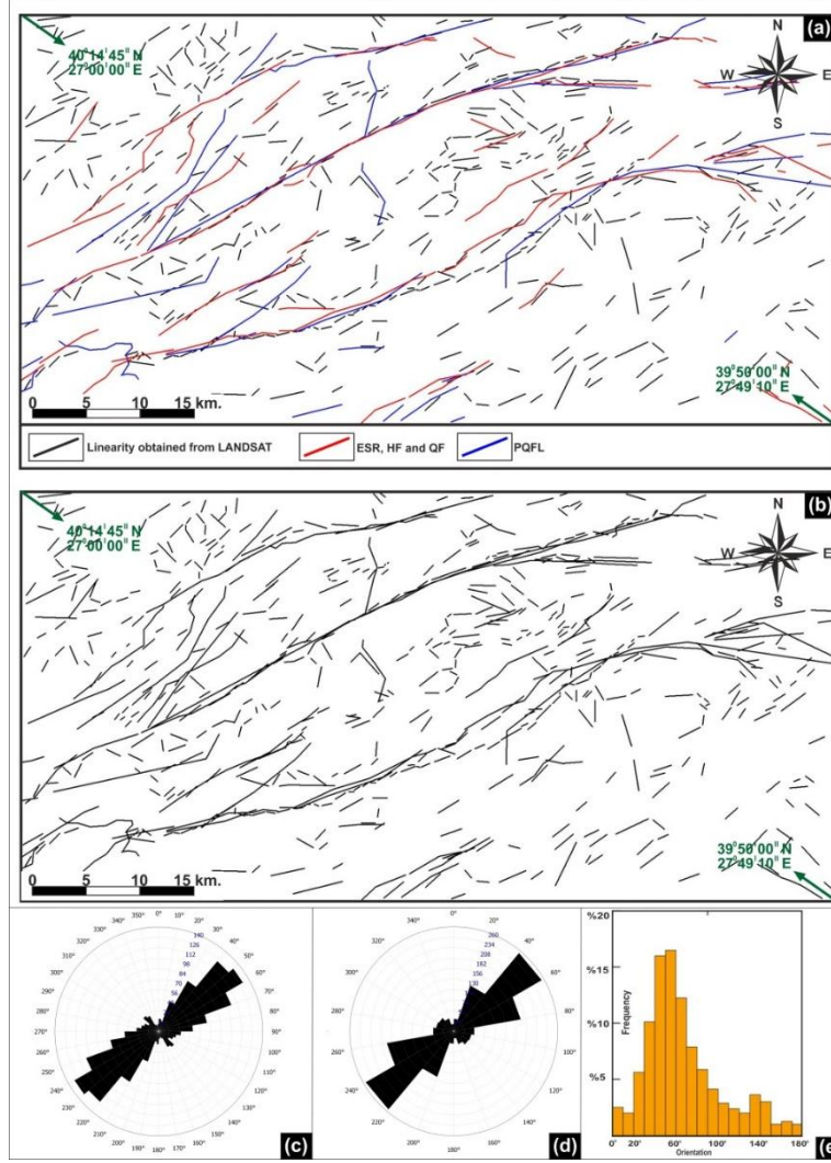
Şekil 9. (a-b) Literatürde gösterilen Olası-Kuvaterner Fayı, çizgisellikler, deprem yüzey kırığı, Holosen Fayı, Kuvaterner Fayı'nın (Emre ve diğ., 2011a, 2011b, 2013) çizgisellik olarak değerlendirilerek harita üzerine işaretlenmesi ve LANDSAT8-OLI uydu görüntüsünden elde edilen çizgiselliklerin ayrı ayrı (a) ve birlikte (b) olacak şekilde tek bir harita üzerinde gösterimi (c) Çizgiselliklerin doğrultularının 10° dilimler halinde gül diyagramında gösterimi (d) Çizgiselliklerin doğrultularının 20° dilimler halinde gül diyagramında gösterimi (e) Çizgiselliklerin doğrultularının 10° dilimler halinde grafik üzerinde gösterimi (0°-90° arası KD doğrultuları; 90°-180° KB doğrultuları gösterir)
