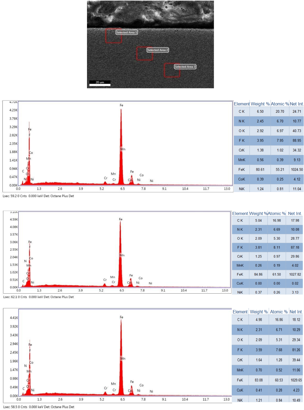
Görsel 3.10. EDS analizi noktaları ve sonuçları
