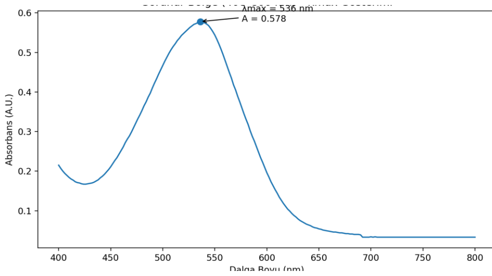
Görsel 1. RR414 boyar maddesinin görünür bölgedeki dalga boyu taraması grafiği
