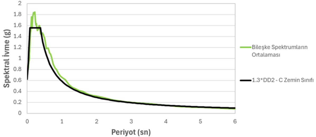
Görsel 5. TBEC 2018'e [26] göre C Zemin Sınıfı için Bileşke Tepki Spektrumlarının Ölçeklendirilmiş Ortalaması
