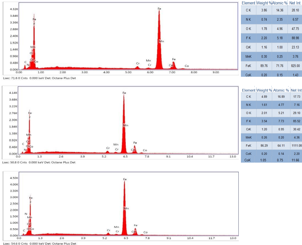
Görsel 3.9. EDS analizi noktaları ve sonuçları
