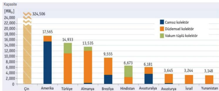
Görsel 4. 2017 yılına kadar dünya çapında güneş enerjisinden sıcak su üretimi teknolojisinde en yüksek kapasiteye sahip ilk 10 ülke ve kolektör tiplerine göre dağılımı (Erdemir & Altuntop, 2018)
