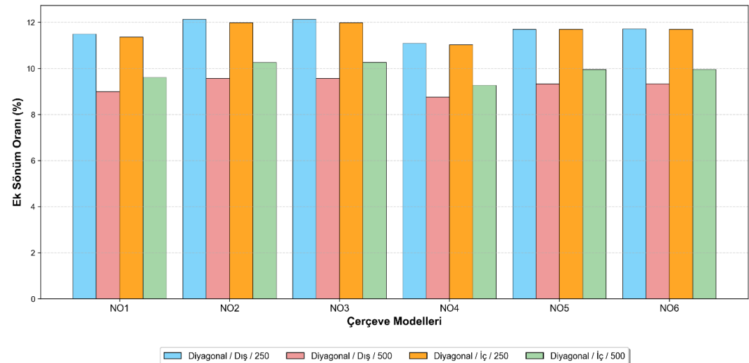
Görsel 13. 15 Katlı Çerçevelerin Ek Sönüm Oranı Grafiği
