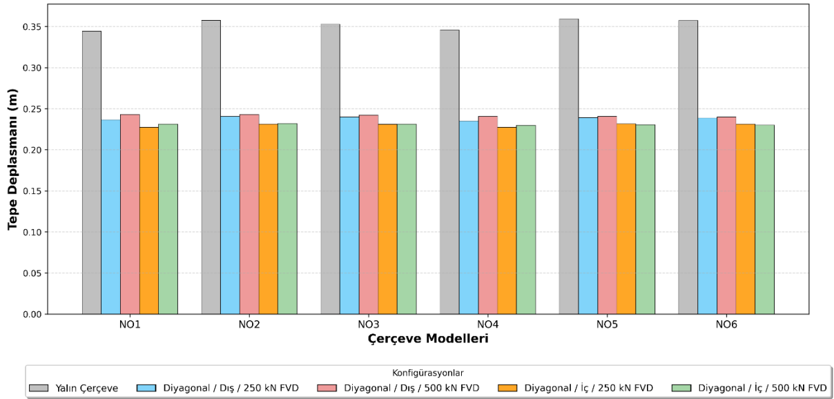
Görsel 9. 15 Katlı Çerçevelerin Tepe Deplasman Sonuçları
