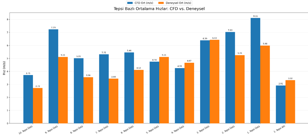
Görsel 10. Tepsi Bazlı Ortalama Akış Hızlarının Karşılaştırması
