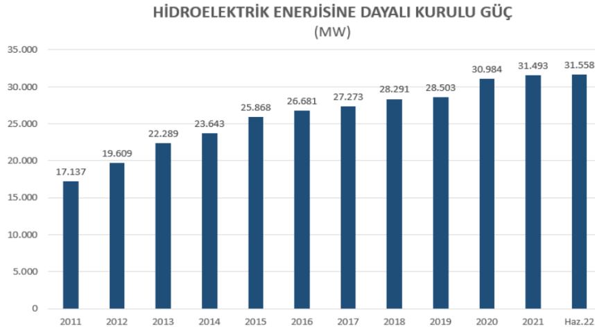
Görsel 1. Türkiye'deki hidroelektrik enerjisine dayalı kurulu güç (MW) (2011-Haziran 2022) (Anonim, 2022)
