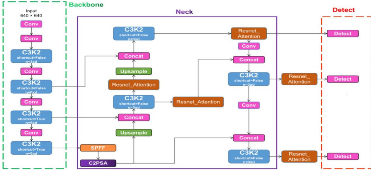
Görsel 1. YOLOv11 Mimarisi [19]
