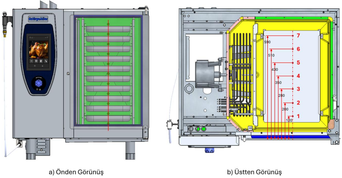
Görsel 3. Ölçüm Noktaları: a) Tepsilerin Üst-Orta Noktalarından Dikey Ölçüm Noktası. b) Her Bir Tepsi için Derinlemesine Yatay Ölçüm Noktaları.
