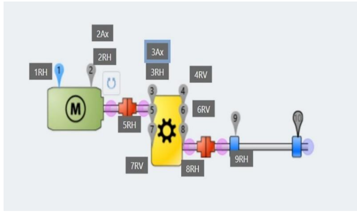
Görsel 1. Kangal Hattı Monoblok İvmeölçer Sensör Yerleşkesi.
