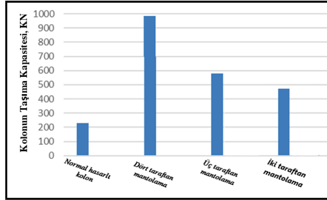
Görsel 3. Farklı taraftan mantolama yöntemlerinin betonarme kolonun taşıma kapasitesi üzerindeki etkiler (Mahmoud ve ark., 2022).
