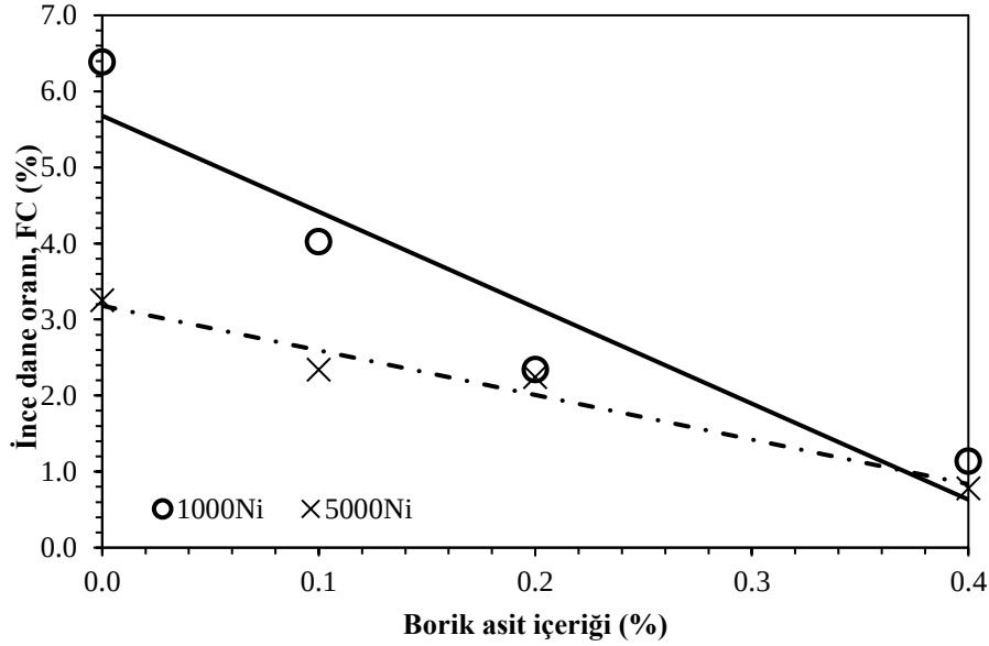
Görsel 6. Borik asit remedasyonunun farklı nikel konsantrasyonlarında ince dane oranı üzerindeki etkisi
