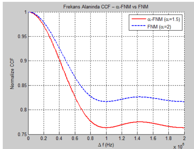
Görsel 2. Frekans Alanı Çapraz İlinti Fonksiyonu Grafiği
