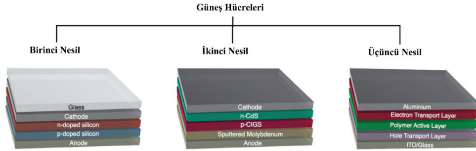
Görsel 12. Nesillere göre hücrelerin şematik gösterimi (Mrinalini, Islavath, Prasanthkumar, & Giribabu, 2019)
