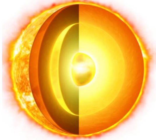
Görsel 1. Güneşin Katmanları, dıştan içeriye doğru; fotosfer, konvektif bölge, ışıma bölgesi ve çekirdek (Bayer, 2018)
