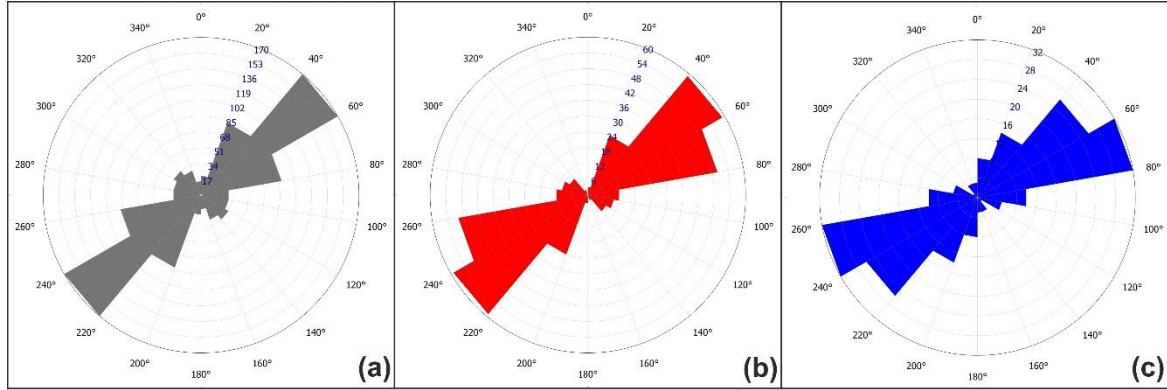
Şekil 10. Çizgiselliklerden elde edilen doğrultuların, 20'lik dilimler halinde gül diyagramı üzerinde gösterimi (a) LANDSAT8-OLI uydu görüntüsünden elde edilen çizgisellikler (b) 1/250.000 ölçekli diri fay haritasındaki aktif unsurlar (c) 1/250.000 ölçekli diri fay haritasındaki aktivitesi kesin olmayan unsurlar ve çizgisellikler
