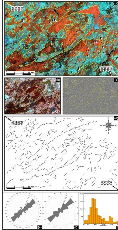
Şekil 6. (a) LANDSAT 8 OLI uydu görüntüsü(RGB: 562) ve üzerinde belirtilmiş çizgisellikler (b) RGB: 562 üzerinde belirlenen çizgiselliklerin, RGB: 632 üzerinde kontrolü (c) RGB: 562 üzerinde belirlenen çizgiselliklerin, pankromatik bantta (Bant 8) 135° yönünde uygulanan 5x5 çekirdek filtresi ile birlikte gösterimi (d) Elde edilen doğrusal yapılar (e) Çizgiselliklerin doğrultularının 10° dilimlerde gösterimi (f) Çizgiselliklerin doğrultularının 20° dilimlerde gösterimi (g) Çizgiselliklerin doğrultularının 10° dilimlerde grafik üzerinde gösterimi (0°-90° arası KD doğrultuları; 90°-180° KB doğrultuları gösterir)
