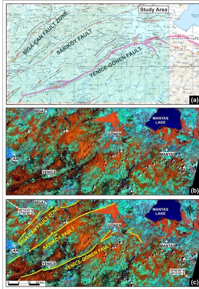
Şekil 5. (a) Çalışma alanında yer alan aktif faylar (Emre ve diğ., 2011a, 2011b) (b) Çalışma alanına ait Local Sigma filtresi ve görüntü keskinleştirme uygulanan RGB:564 uydu görüntüsü (c) Bu uydu görüntüsü üzerine çizilmiş ana faylar
