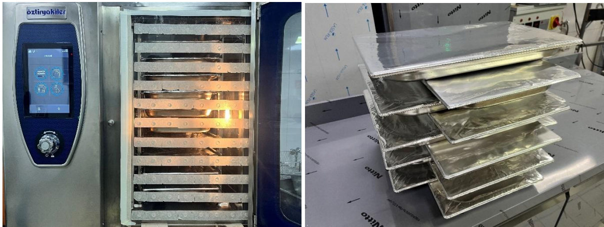
Görsel 1. Endüstriyel Pişirme Fırını ve Alüminyum Folyo ile Kapatılmış GN 1/1 Gastronom Küvetler
