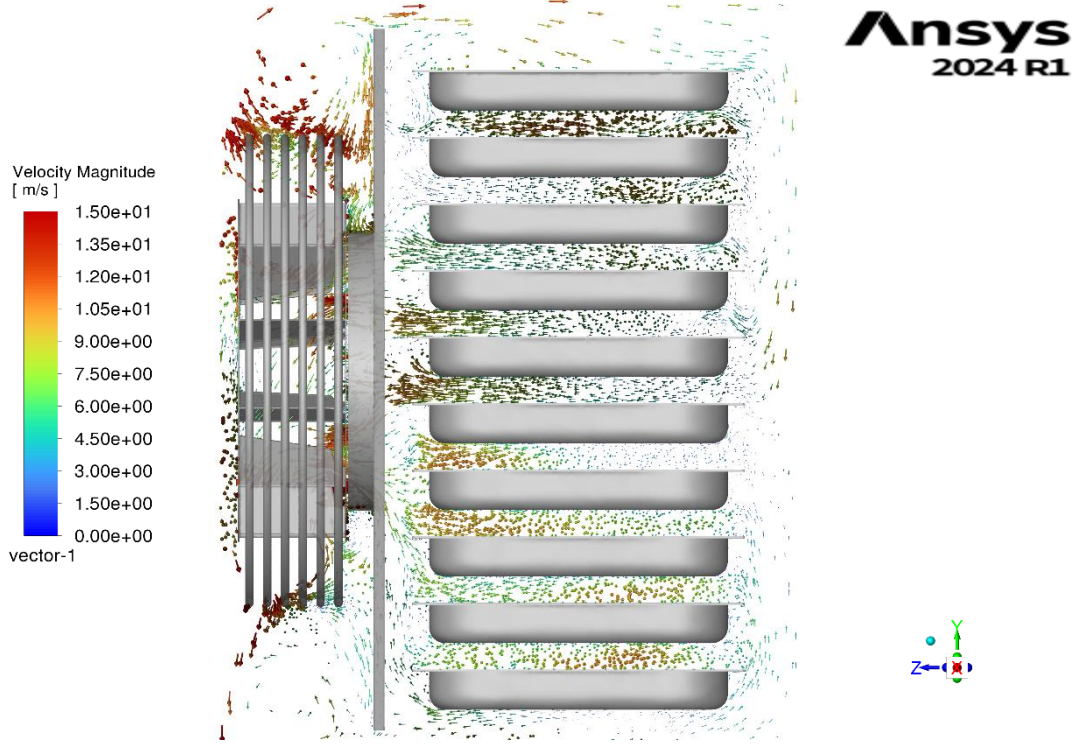
Görsel 8. CFD Simülasyonundan Elde Edilen YZ Eksinindeki Akış Çizgileri
