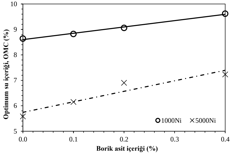
Görsel 10. Borik asit remedasyonunun farklı nikel konsantrasyonlarında optimum su içeriği üzerindeki etkisi
