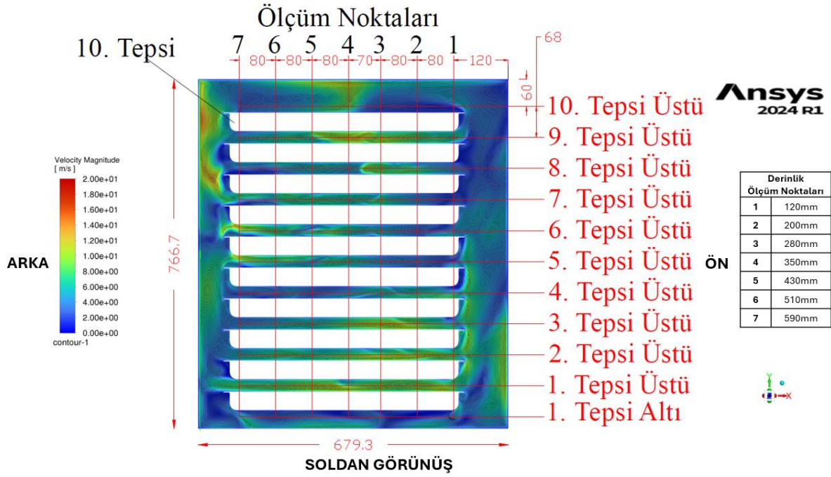
Görsel 6. CFD'den Elde Edilen Akış Hızlarının Okuma Noktaları (Ön: Kapı Tarafı)
