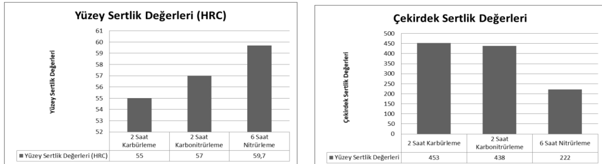
Görsel 3.1. Yüzey ve Çekirdek sertlik değerleri.
