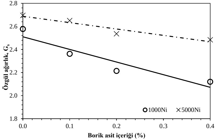
Görsel 7. Borik asit remedasyonunun farklı nikel konsantrasyonlarında özgül ağırlık üzerindeki etkisi
