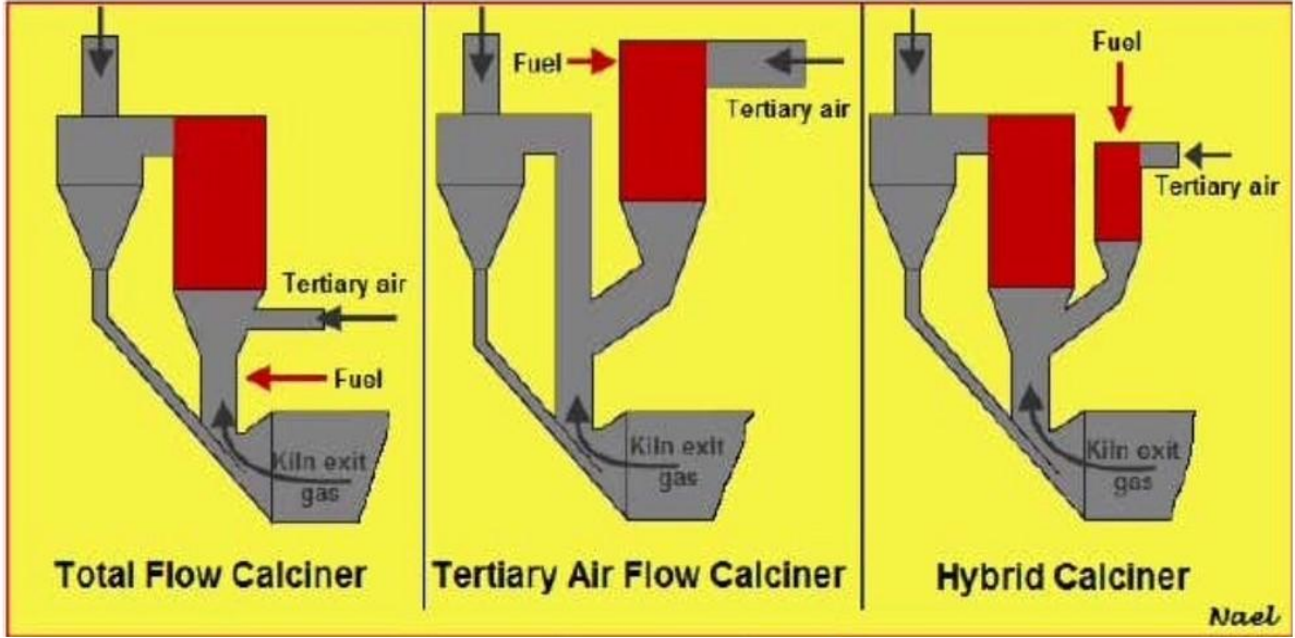
Görsel 3. Önkalsinatör tipleri
